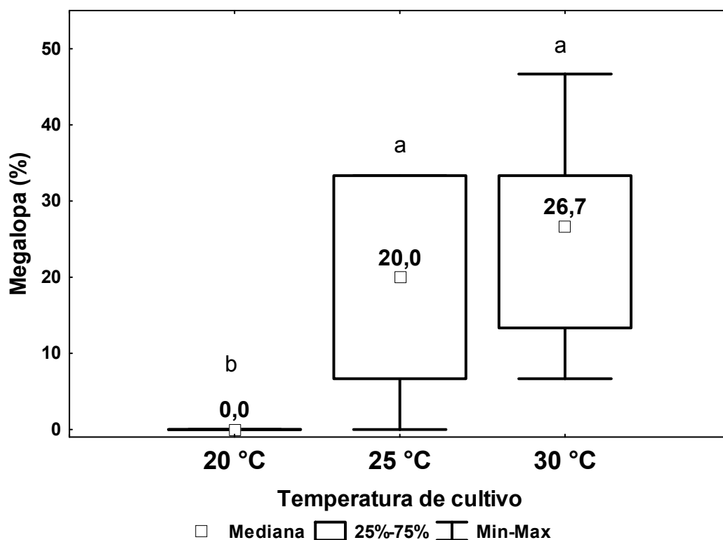
Figura 6 Taxa de sobrevivência até o estágio de megalopa das larvas de U. cordatus cultivadas na temperatura de 25 e 30(±1)°C. Letras iguais identificam tratamentos que não apresentaram diferenças significativas ao nível de 5% conforme teste de Dunn a posteriori .
